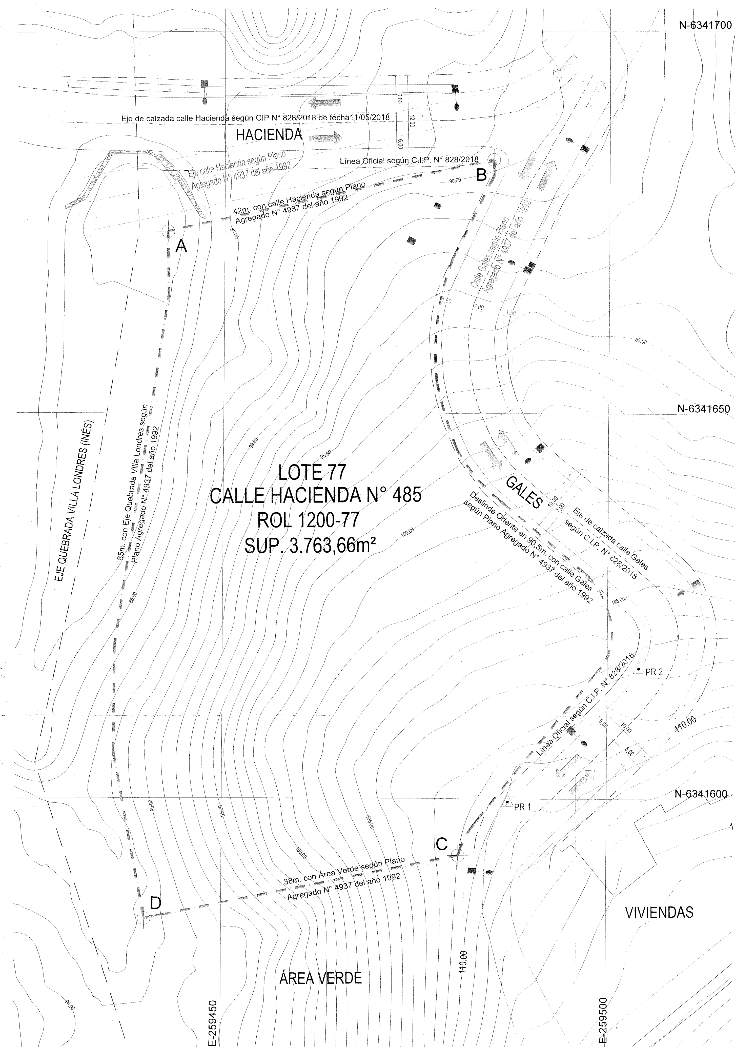
PLANO SITUACIÓN EXISTENTE ESCALA 1:250
