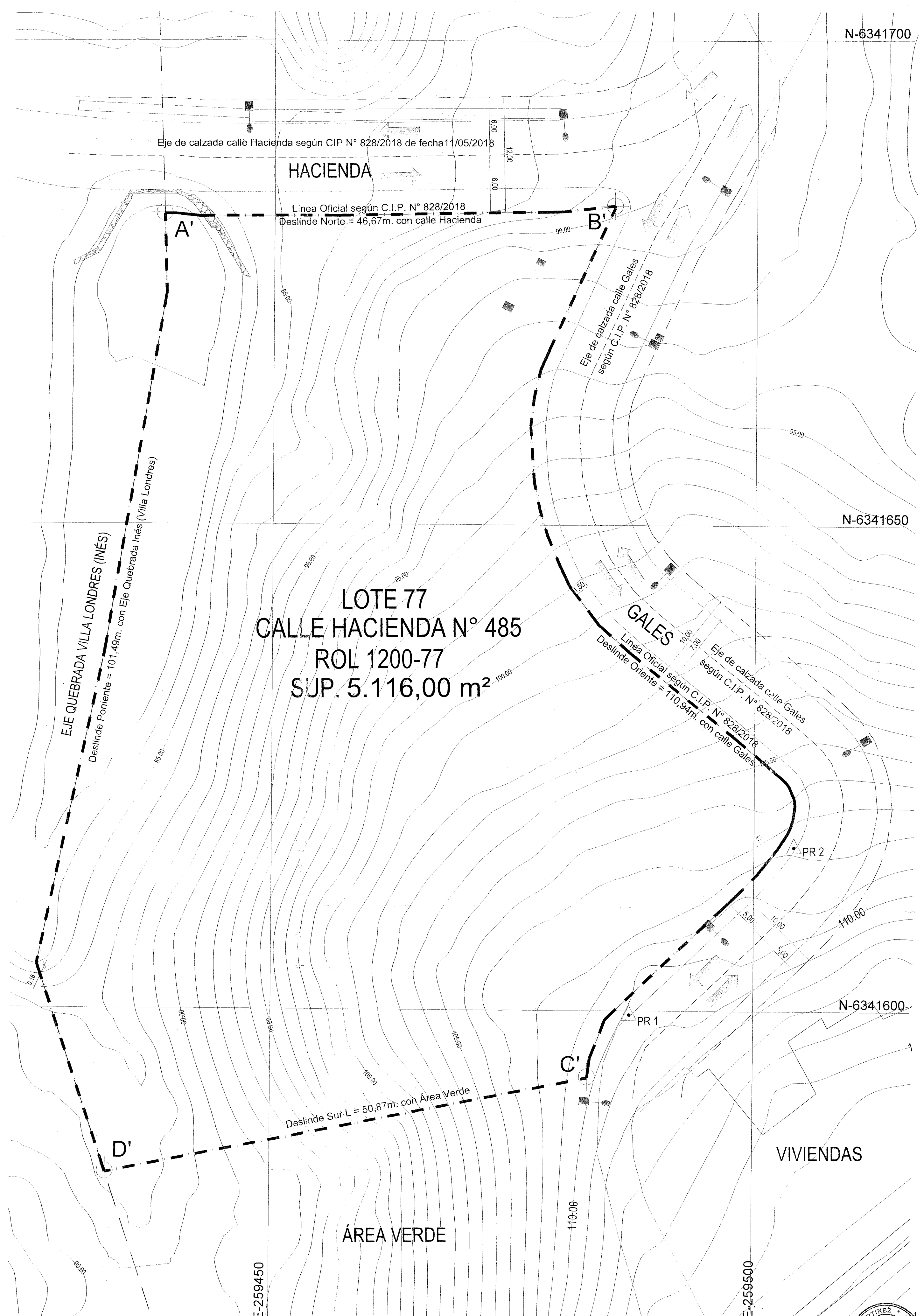
PLANO SITUACIÓN MODIFICADA ESCALA 1:250
